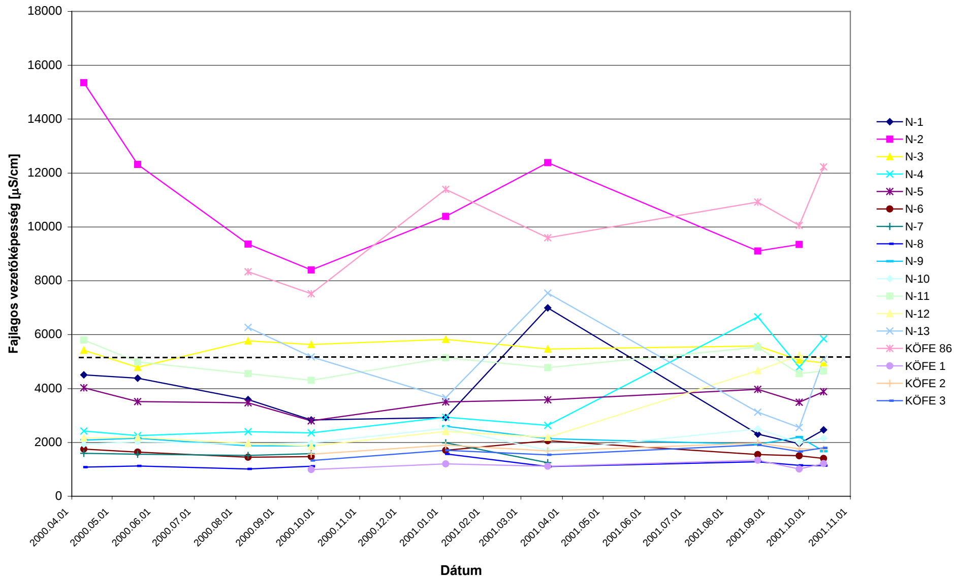
Fajlagos vezetőképesség időbeli változása az egyes monitoringkutakban a kármentesítés során (2000. 04. 10 - 2001. 10. 12.)
